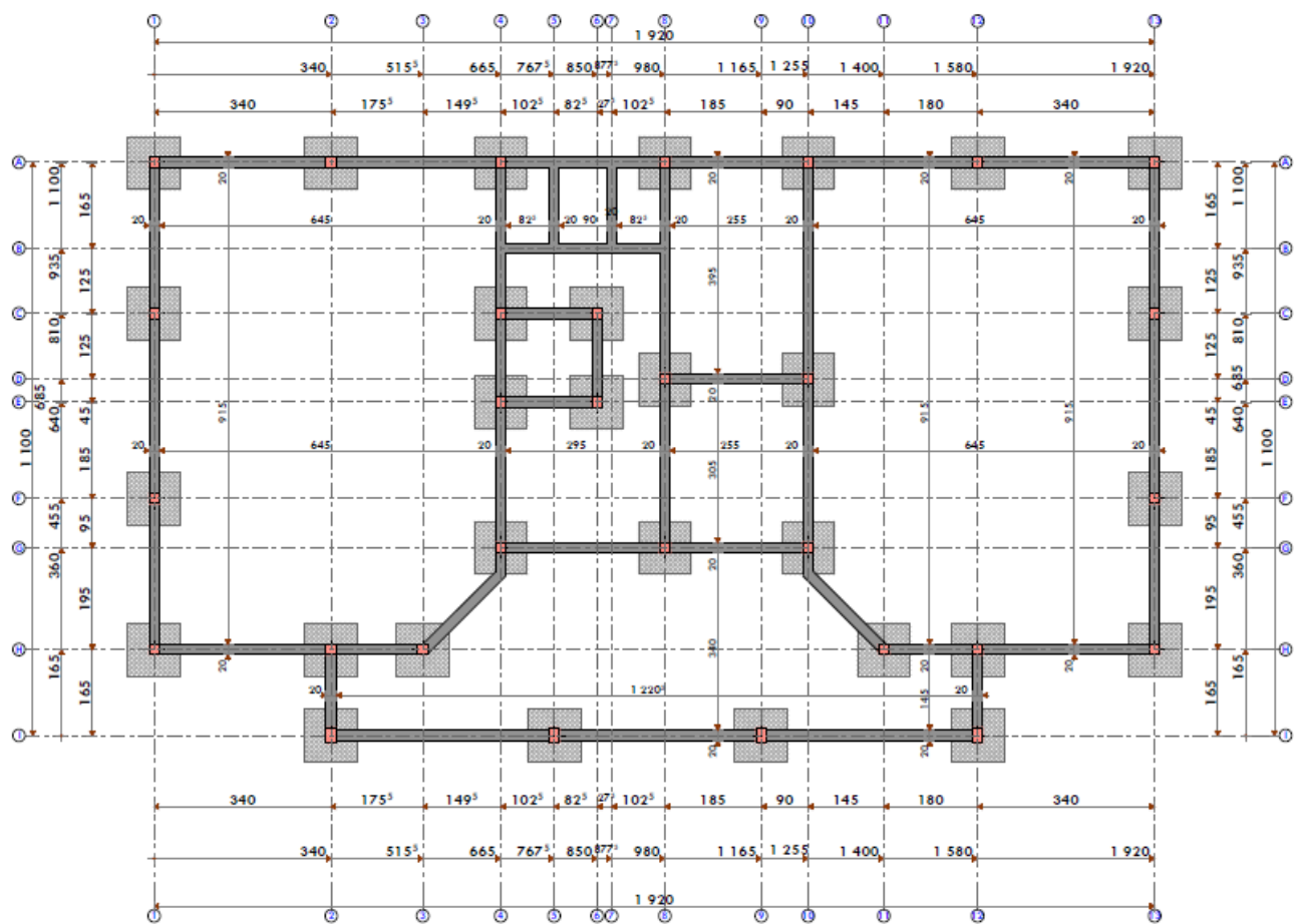
PLAN DE FONDATION - FOUNDATION PLAN
